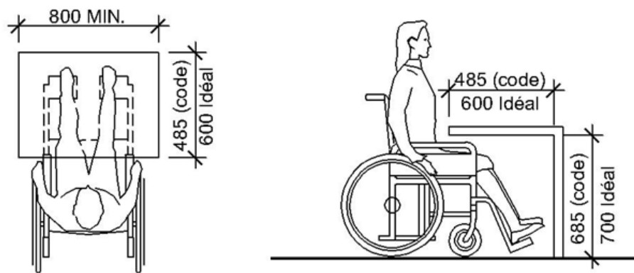
Illustration des dégagements minimaux (Code) et souhaitables
